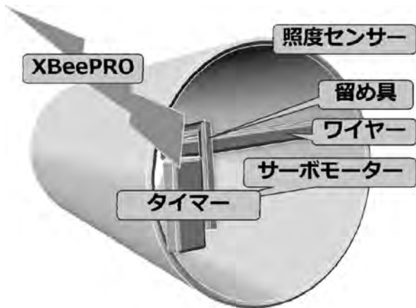
図6 キャリアの開放機構の説明図
