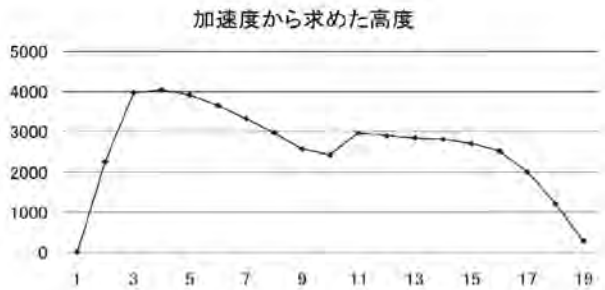
図12 加速度から求めた高度(縦軸は高度[m], 横軸は時間[分])
